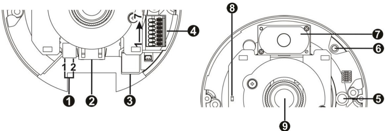
Kamera NVIP-12DN7023V/IR-1P
